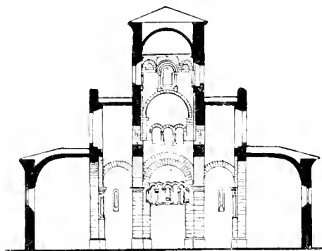
Église de Germiny-les-Prés. — Coupe.
